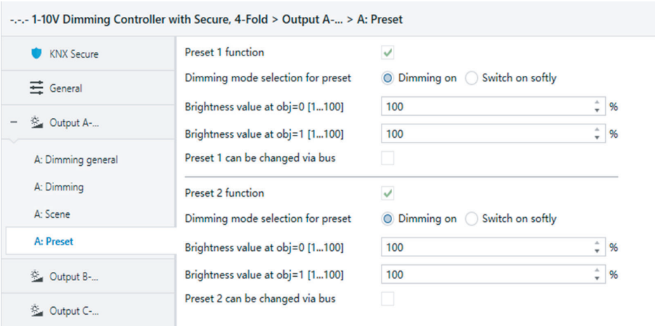
Fig. 5.5.4 parameter window "X: Preset"
