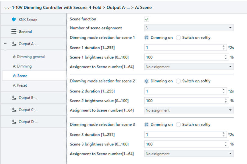
Fig. 5.5.3 parameter window "X: Scene page"
