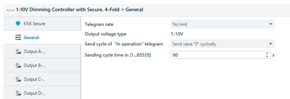
Fig. 5.2 Parameter window "General"
