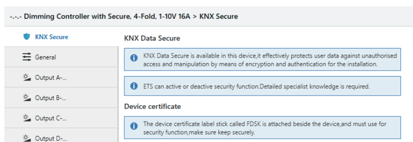
Fig.5.1 (1) "KNX Secure" parameter window
