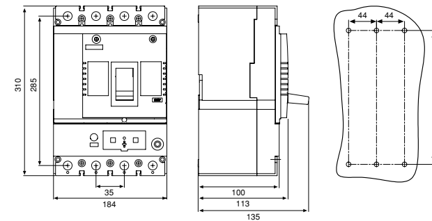
VMR4-SN2
