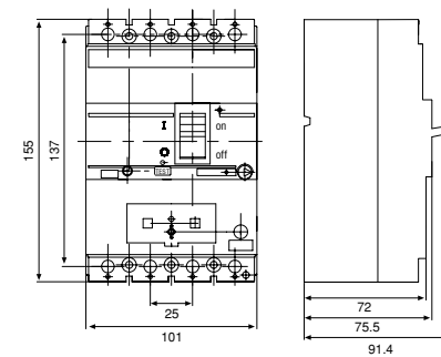
VMR4-SN2
