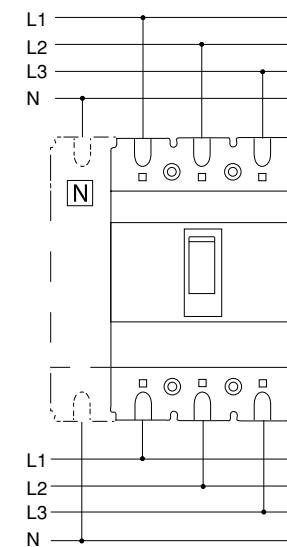
4 Kutuplu Kompakt Şalter Bağlantı Şeması
