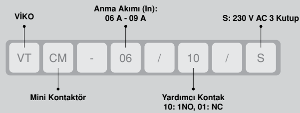
Mini Kontaktörler
