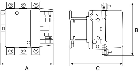
VTC 630 - 800
