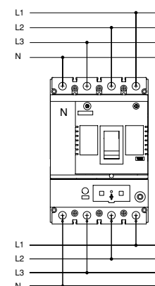
4 Kutuplu Kompakt Şalter Bağlantı Şeması
